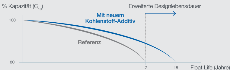
Labortests zeigen, dass das Kohlenstoff-Additiv zu einer Verlängerung der Lebensdauer um bis zu 3 Jahre führt
